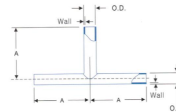
Reducing Tee, Long (Tube) 异径三通 ASTM A269/A270
