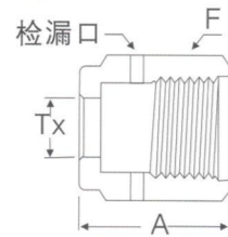
Nut Female 内螺纹螺母
