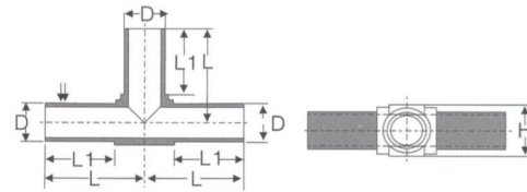
Equal Tee 同径三通
