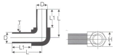
90° Elbow 弯头
