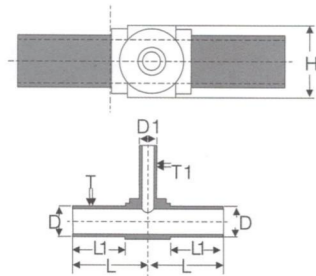
Reducing Tee 异径三通
